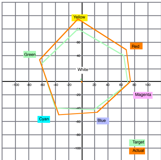
Comparison Target Color Space / Actual Color Space
